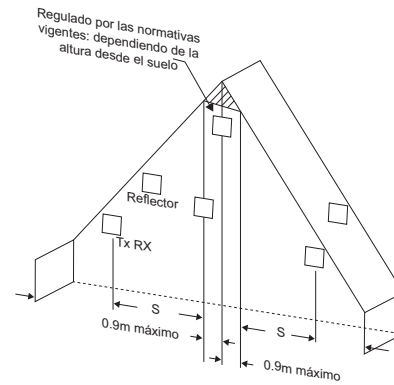
Figura 7-4: Techo inclinado (de tipo pico)
