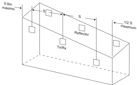
Figura 7-3: Techo inclinado (de tipo cobertizo)
