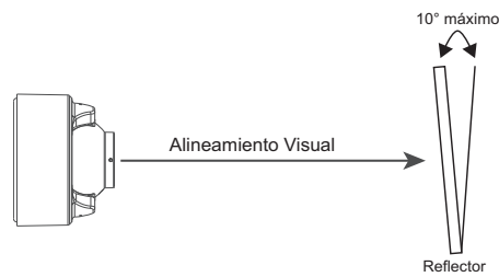
Figura 9-3: Instrucciones de montaje del reflector
