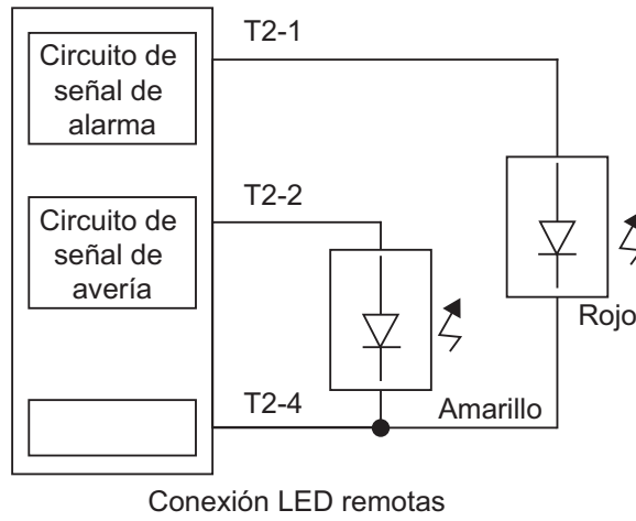
Figura 11-5: Diagrama de cableado (LED remotos)
