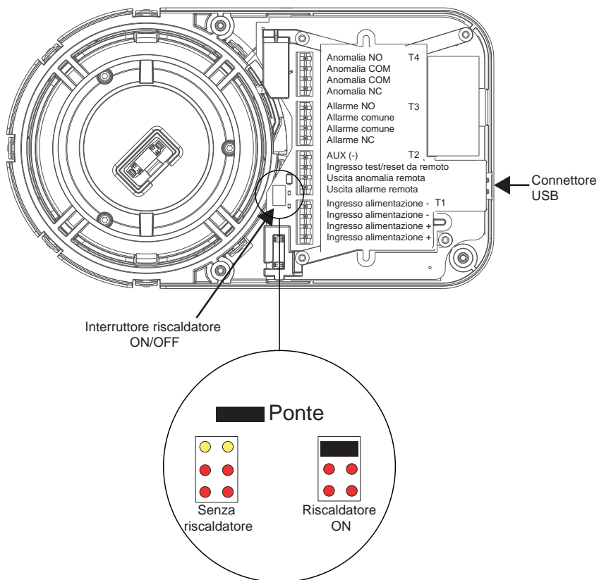
Figura 12-3: Connessioni elettriche presso il rivelatore
