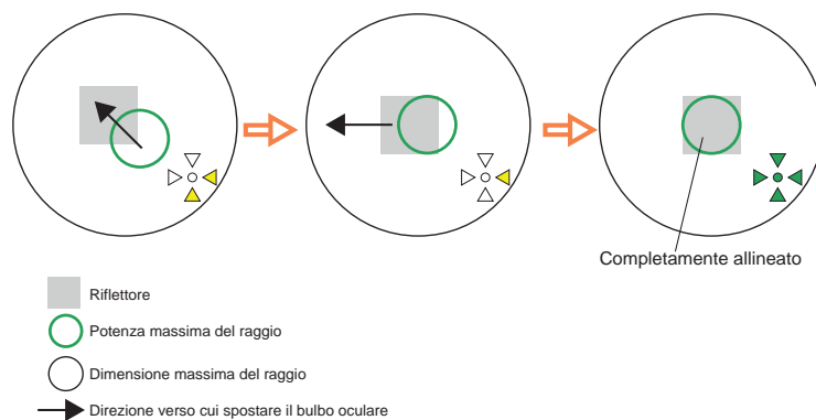
Figura 13-4: Guida a colori del set frecce per l'allineamento
