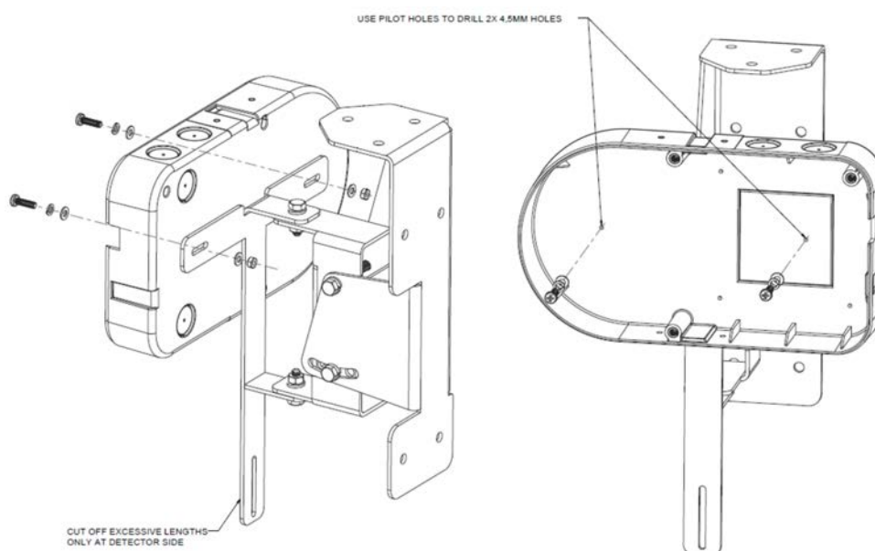
Figura 12-1: Linee guida per il montaggio del rivelatore
