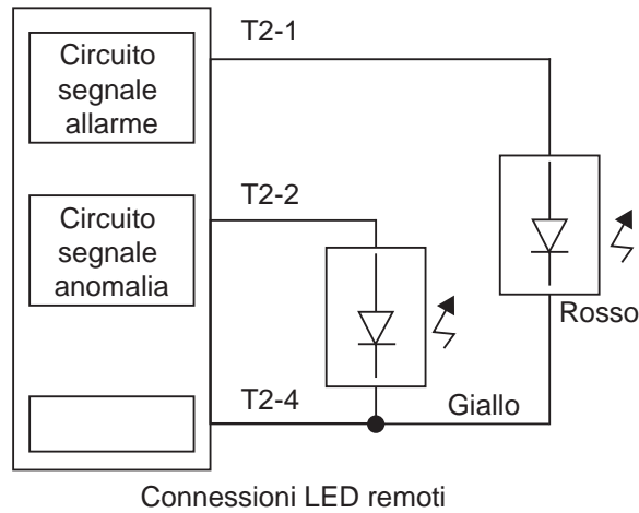
Figura 12-5: Schema elettrico (LED remoti)
