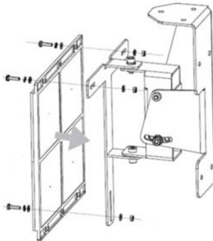
Figura 10-2: Linee guida per il montaggio del riflettore
