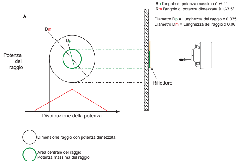
Figura 13-2: Distribuzione potenza raggio
