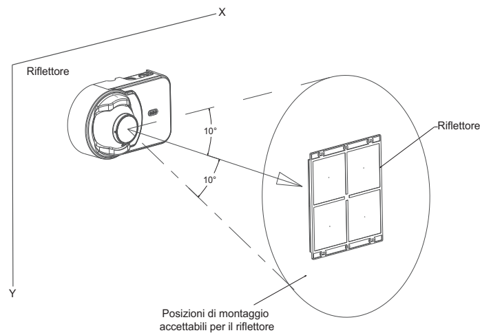
Figura 10-1: Linee guida per il montaggio del riflettore
