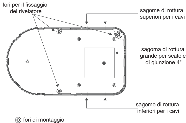
Figura 10-4: Fori di guida per il montaggio
