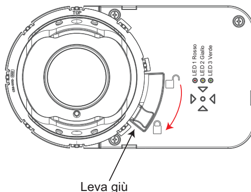
Figura 13-5: Bloccare e assicurare il bulbo oculare
