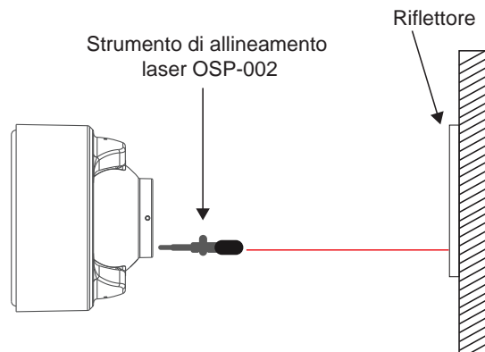
Figura 13-1: Allineamento grezzo
