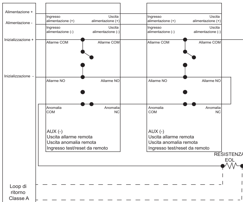
Figura 12-2: Schema elettrico
