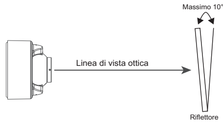
Figura 10-3: Linee guida per il montaggio del riflettore
