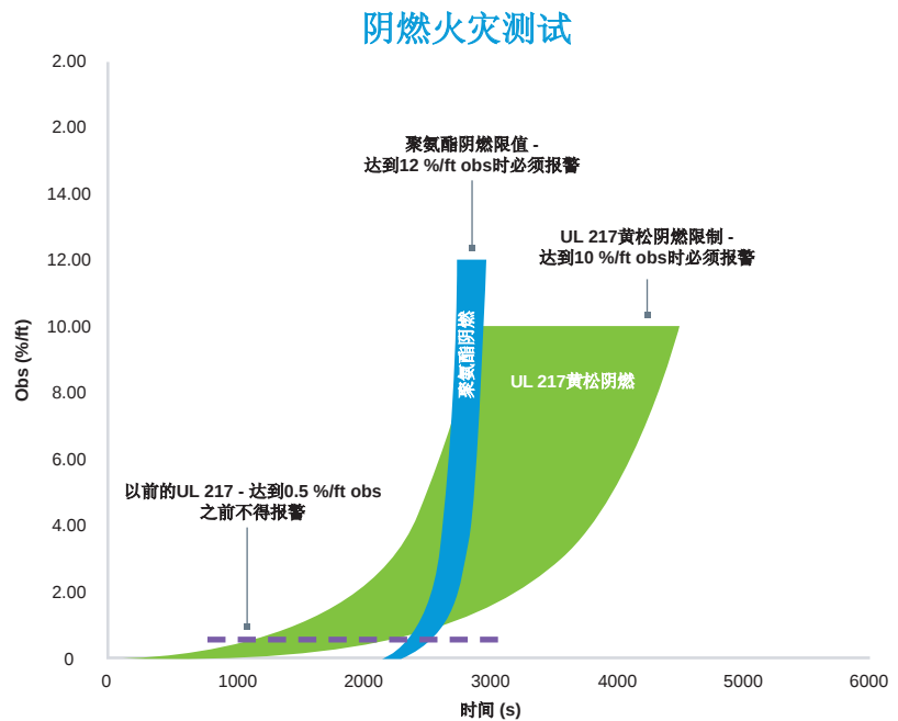
图1 - 聚氨酯和黄松的阴燃比较 1
