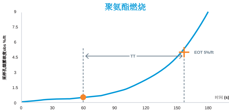
图3 - 特殊应用聚氨酯燃烧测试
