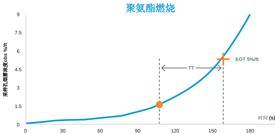
图2 - 开放区域聚氨酯燃烧测试
