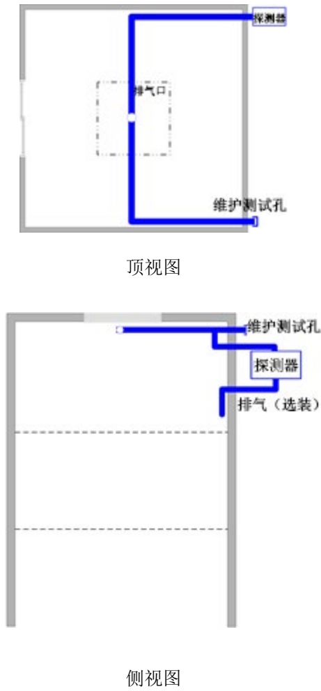
图1: 电梯井消防 (≤4层)
