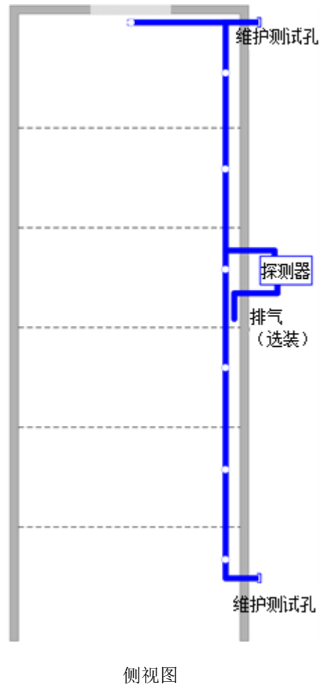
图2: 电梯井消防 (>4层)
