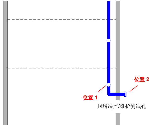
图 5: VESDA ASD 管网 - 维护
