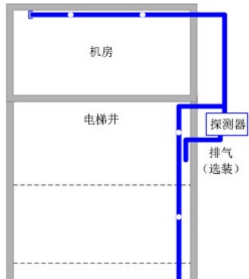
图4: 机房/电梯井消防
